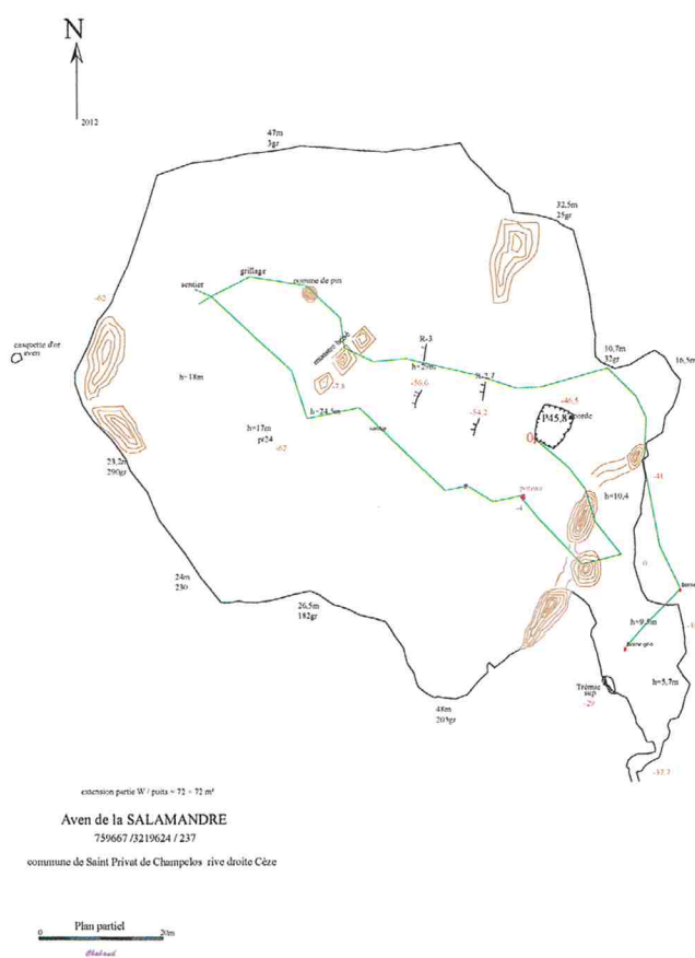
Ci-dessus: topo de Michel Chabaud Ci-dessous: plan de la grotte transmis par Michel Wienin
