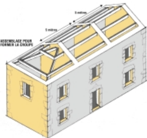
Toiture à trois pentes
