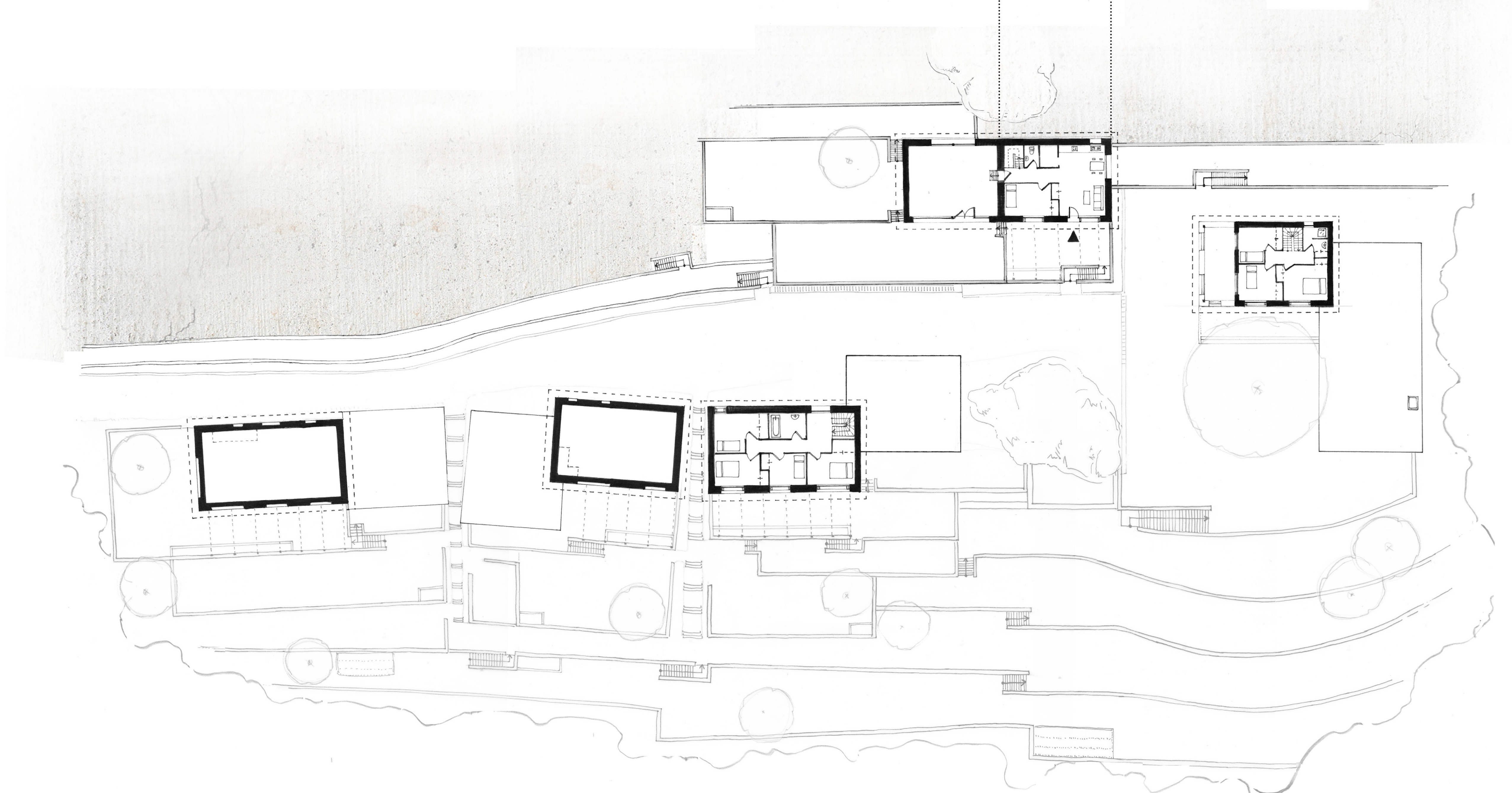
PLAN R+1 éch. 1/200
