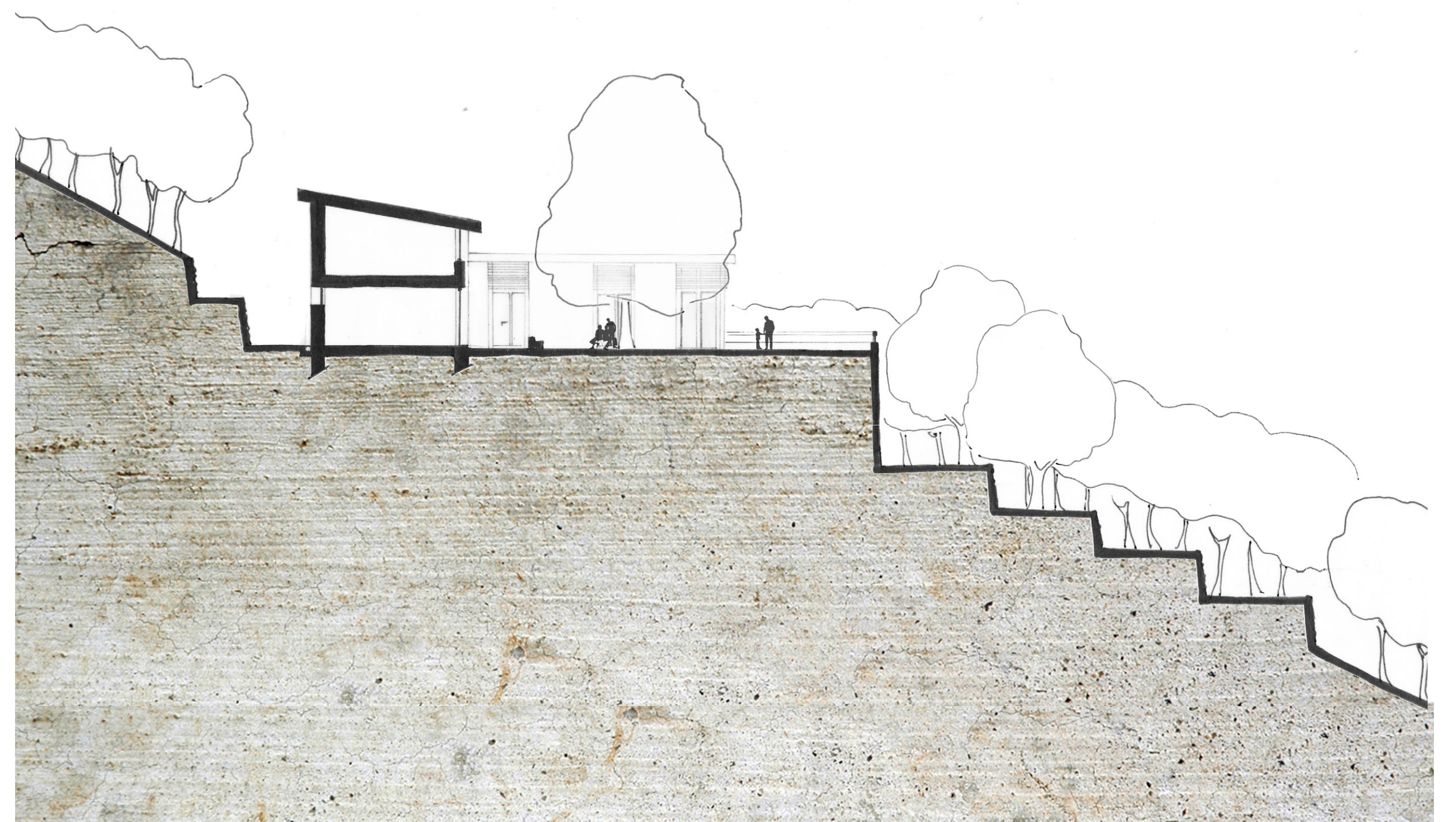
COUPE DD' éch. 1/200
