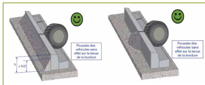
Figure 31 : Calage par solin continu (à gauche) et par épaulement (à droite) (source : Cérrib, document 152.E_v3)
