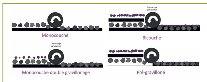
Figure 23 : Schéma de réalisation de différents types d'enduits (Dessin de C. Houel)
