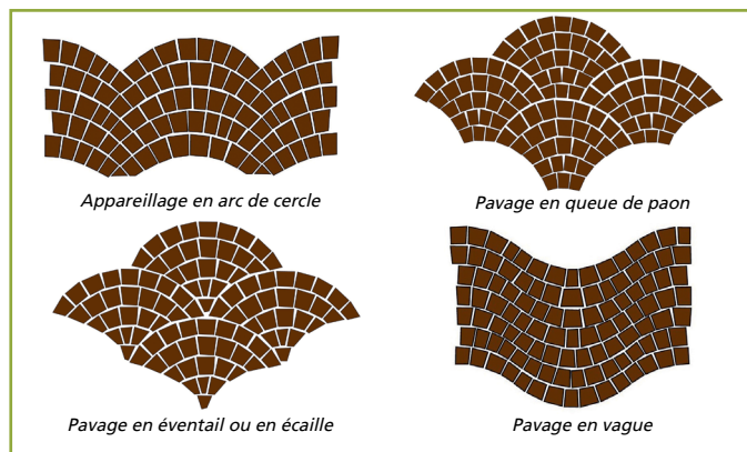
Figure 8 : Exemples d'appareillages (Dessin de C. Houel)
